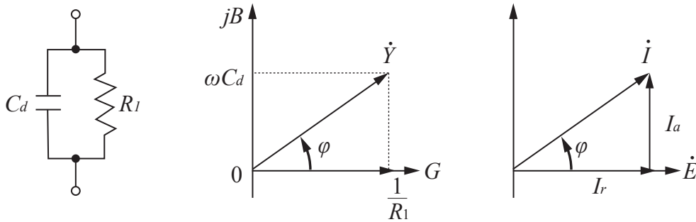
振动子共振时的矢量图
